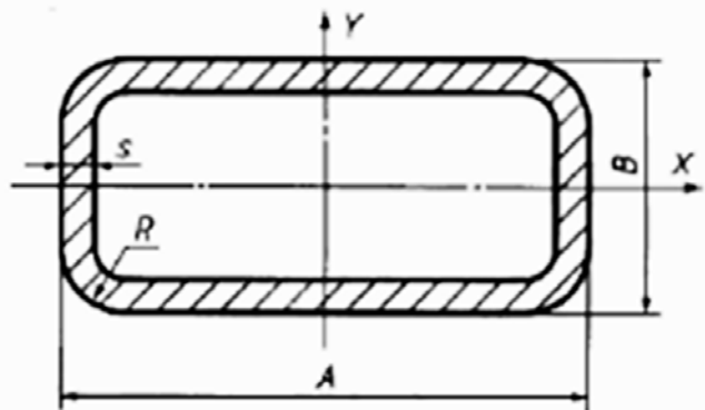
Сортамент профиля
