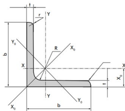
Сортамент профиля
